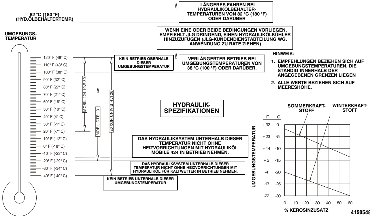
Abbildung 6-3. Motorbetriebstemperatur-Spezifikationen - Deutz - Blatt 2 von 2
