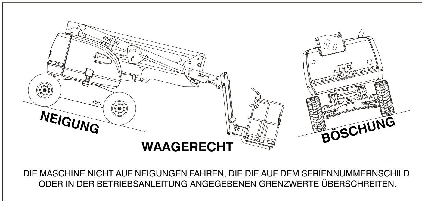
Abbildung 4-3. Neigung und Böschungen
