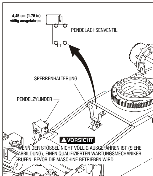
Abbildung 2-5. Tägliche Sichtkontrolle - Blatt 3 von 3
