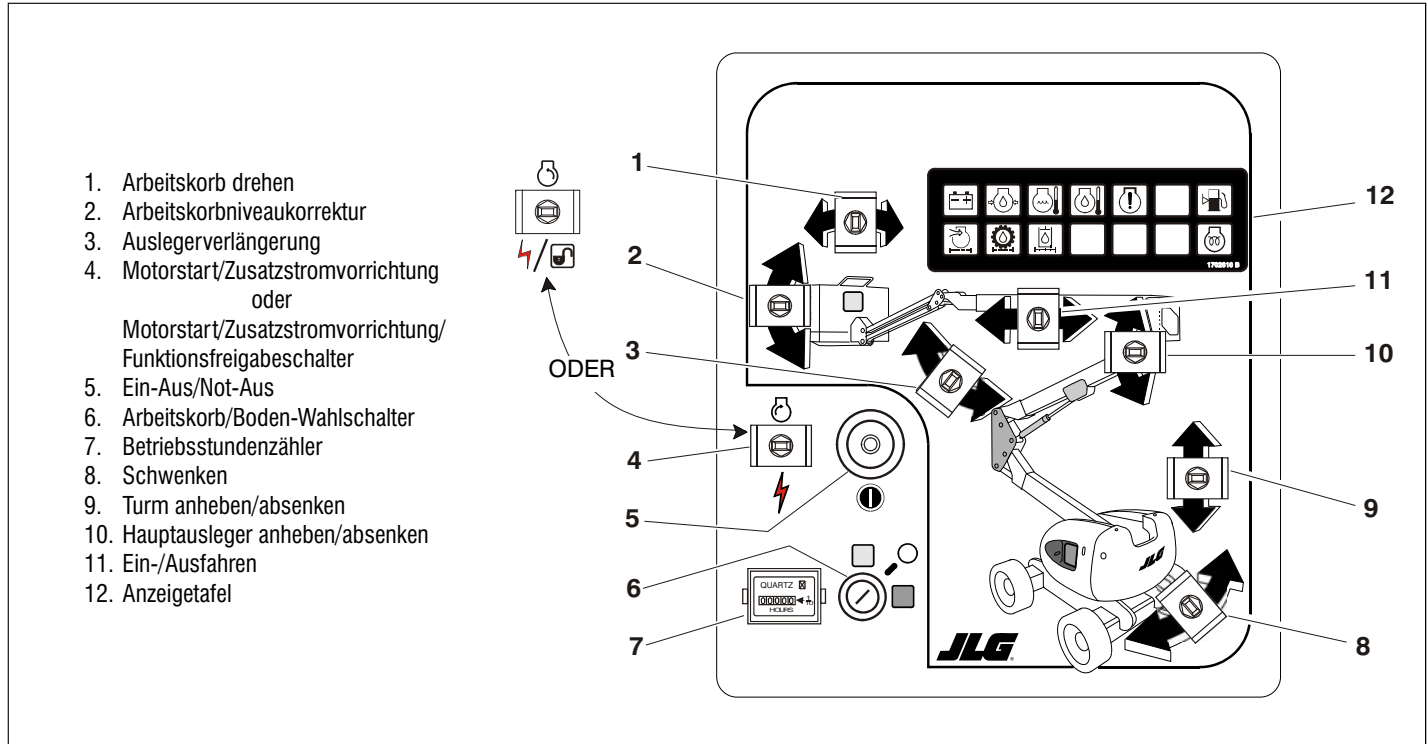
Abbildung 3-1. Boden-Bedienpult - AJ-Modelle
