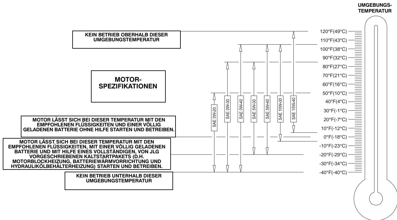
Abbildung 6-6. Motorbetriebstemperatur-Spezifikationen - Caterpillar - Blatt 1 von 2
