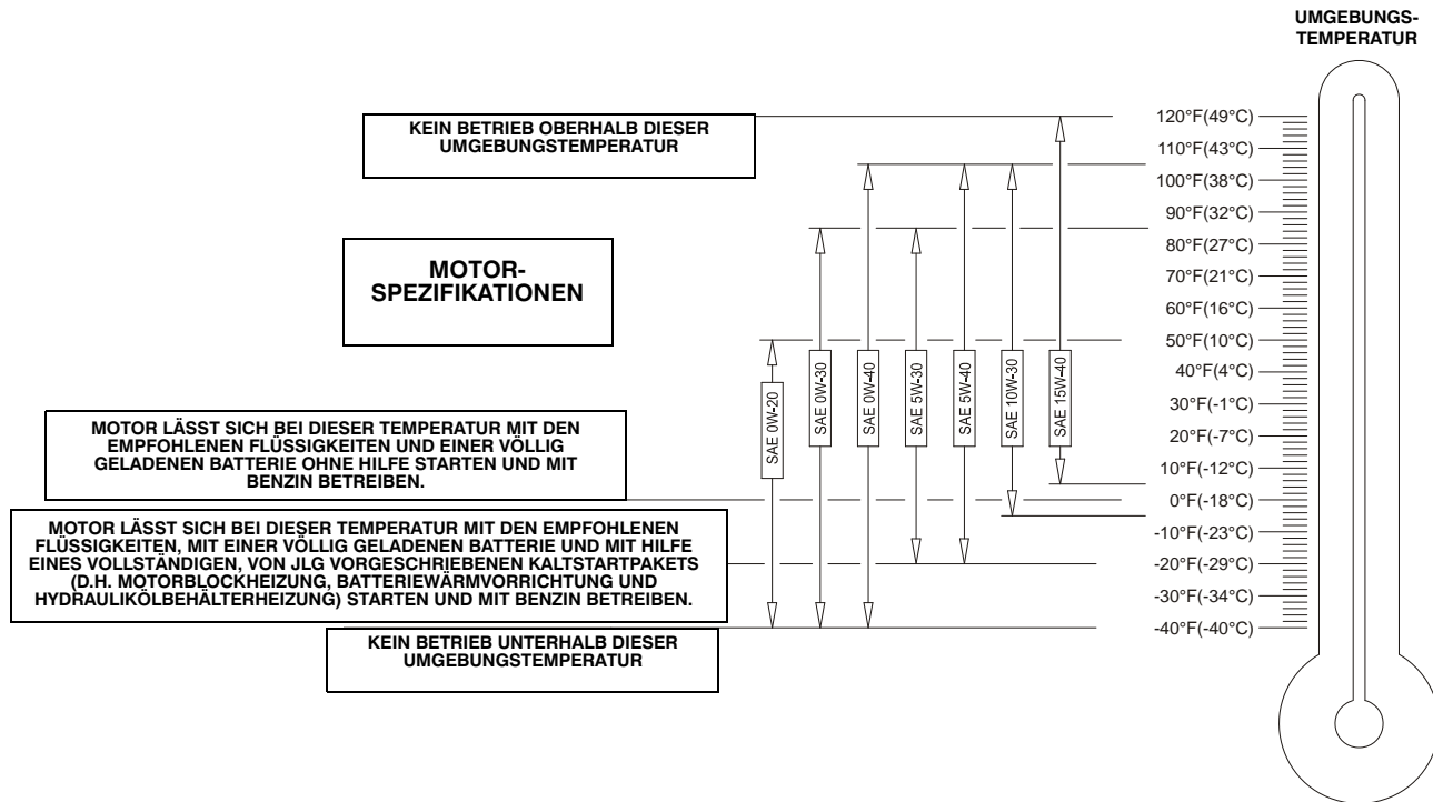
Abbildung 6-10. Motorbetriebstemperatur-Spezifikationen - Perkins - Blatt 1 von 2
