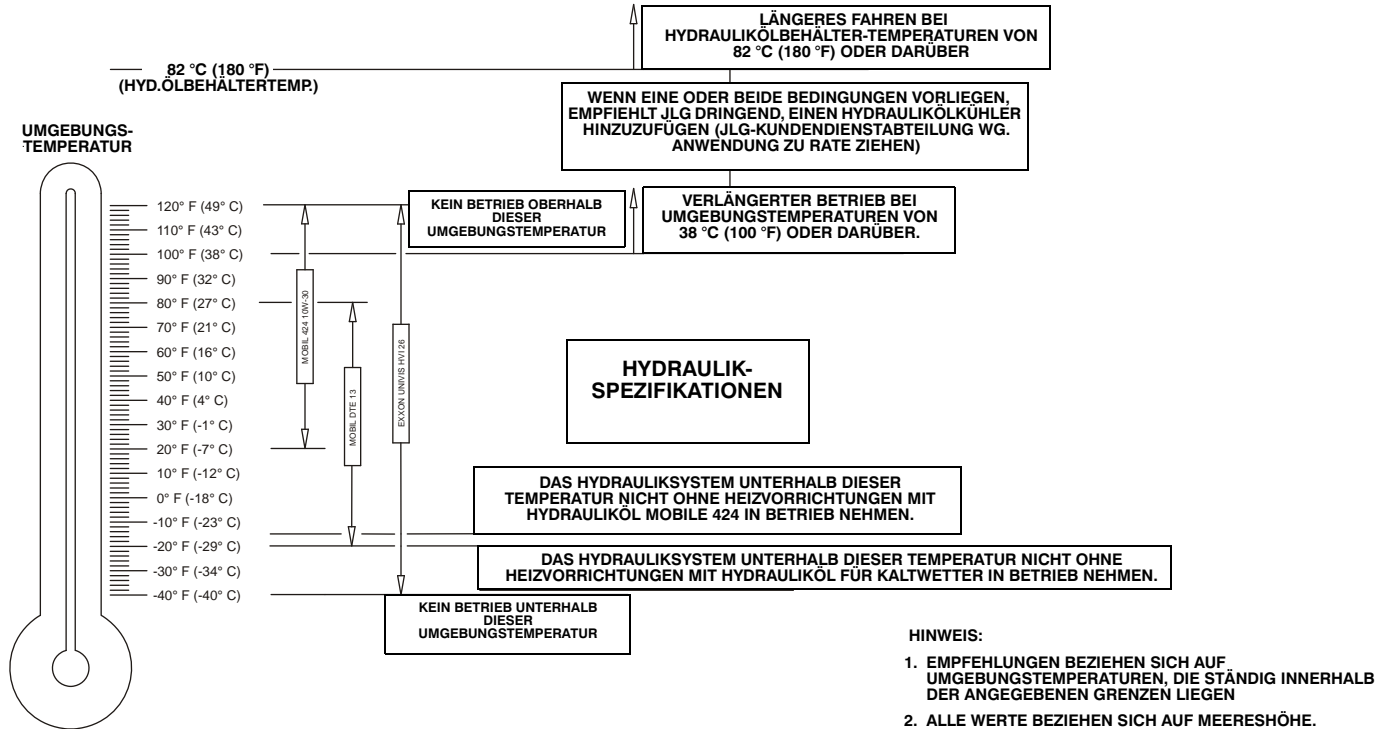
Abbildung 6-11. Motorbetriebstemperatur-Spezifikationen - Perkins - Blatt 2 von 2
